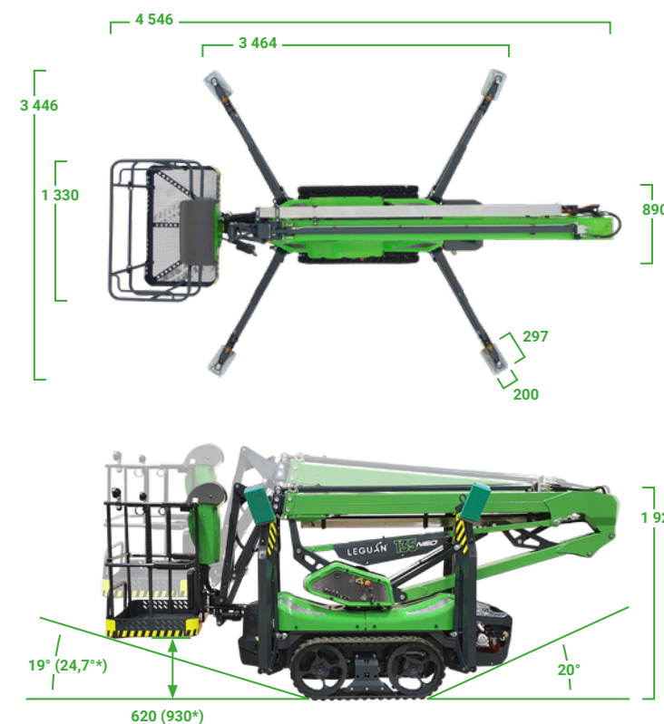
Mått i millimeter. *En förhöjd körposition (EDP) maximerar värdet. **En förhöjd körposition (EDP) maximerar värdet.
