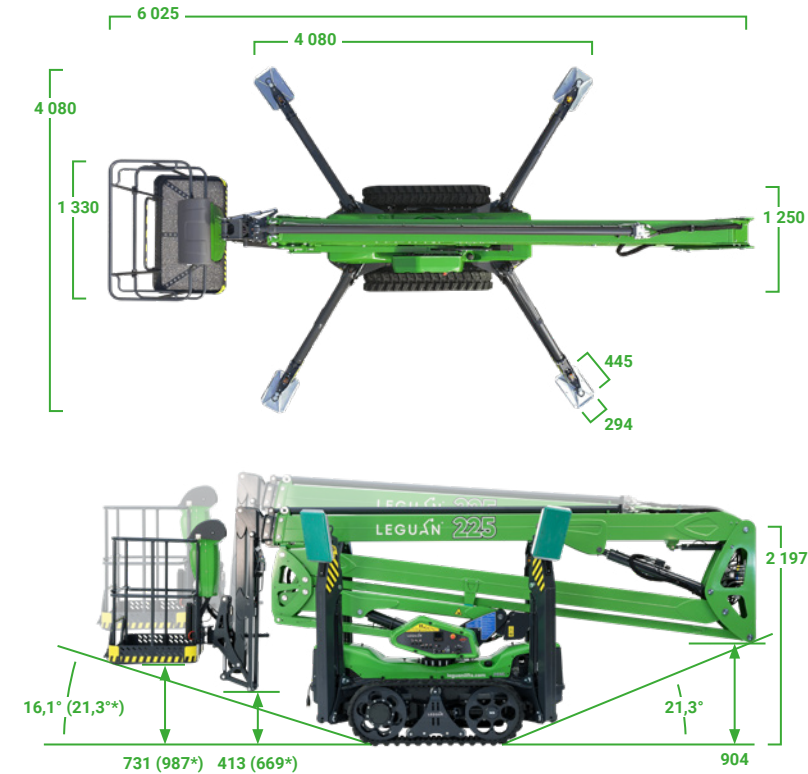
Mått i millimeter. *En förhöjd körposition (EDP) maximerar värdet.
