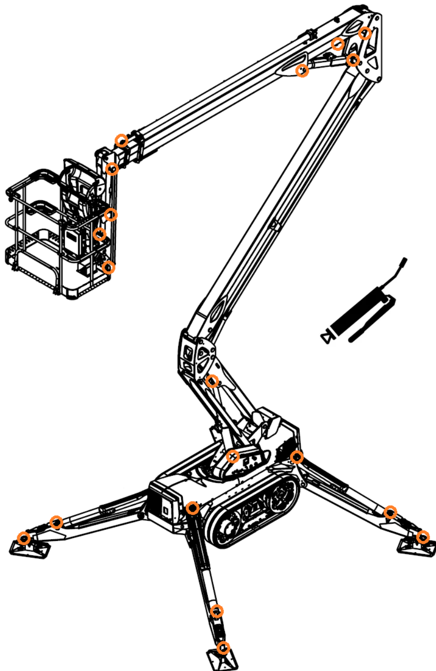
Figur 15. Smøreskjema
