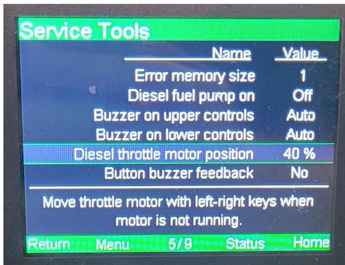
Figur 29. Gasspjeldmotorens posisjon
