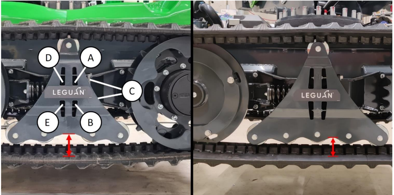
Figur 12. Justering av beltestramming
